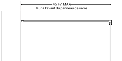
Dimensions de la barre de support
