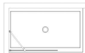
Installation de la barre de support du mur latéral jusqu'au panneau fixe
