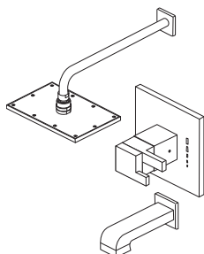
GARNITURE TEMPASSURE™ POUR BAIGNOIRE-DOUCHE THERMOSTATIQUE
